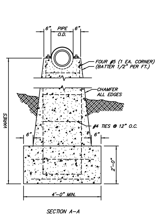
CONCRETE PIPE SUPPORT N.T.S. SS.3.1
